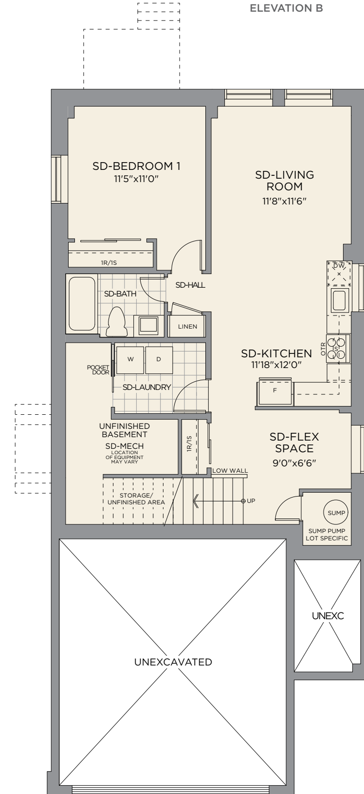
ELEVATION B
